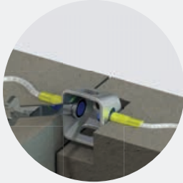
Abb. BT-Spannschloss® (Verbindung von Betonfertigteilen)
