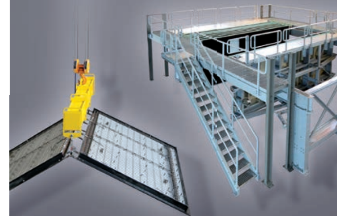
Die patentierte Batterie- und Schmetterlingsschalung von BT innovation
